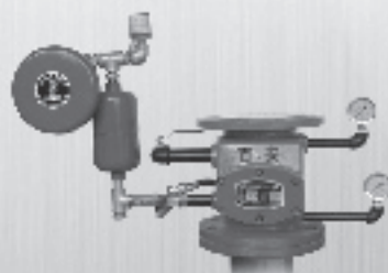
罐式报警阀
